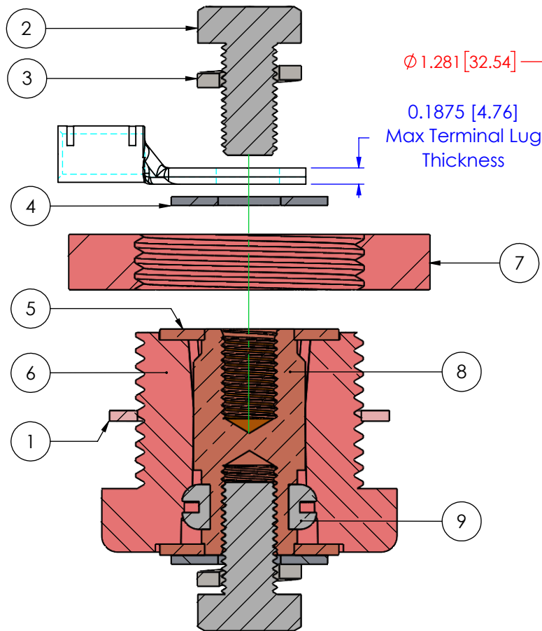
SECTION A-A
